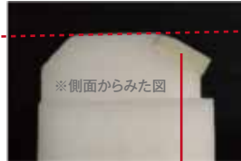
※側面からみた図 摩耗した分離パッド。 頂点が摩耗し、プラスチック部品と 同じ高さまで擦り減っている。交換が必要。
